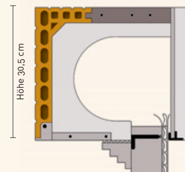
WDVS-Ausführung für Vollwärmeschutzsystem
