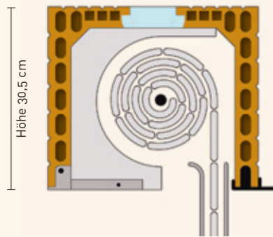
Universal-Ziegel-Raffstore-Rollladenkasten bzw. Ziegel-Raffstore-kasten für Mauerstärke bis 50 cm
