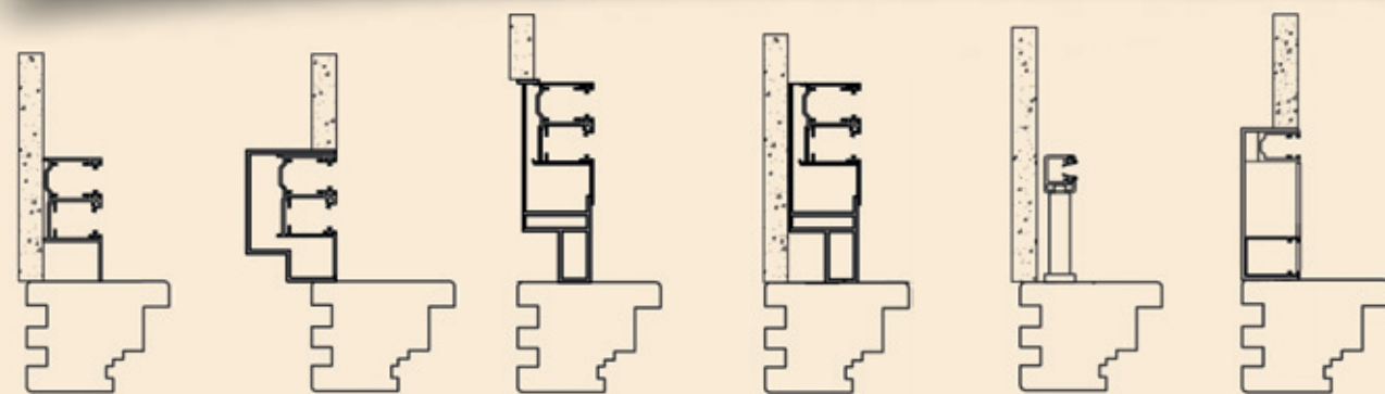
Doppelführungsschiene für Rollläden und Insektengitter
