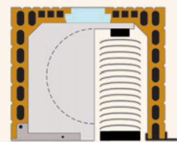
Universal-Ziegel-Raffstore-Rollladenkasten bzw. Ziegel-Raffstore-kasten für Mauerstärke bis 50 cm
